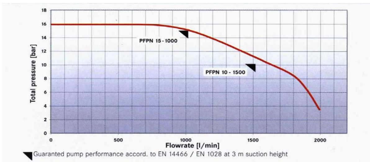
Rosenbauer Fox III tuottokäyrä mitattuna 3 metrin imukorkeudella
